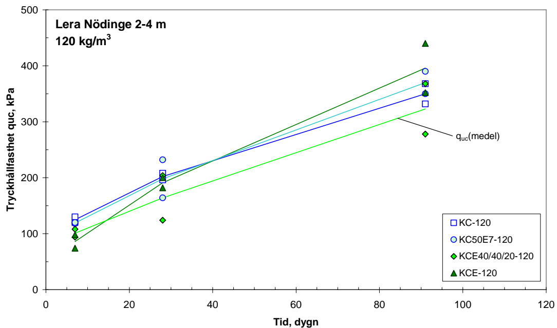
Figur 8.5. Uppmätt hållfasthetstillväxt med tiden efter inblandning för stabiliserad jord från 2-4 m djup i Nödinge. Bindemedelsmängd (a) 90 kg/m 3 och (b) 120 kg/m 3 . Benämning, se tabell 7.2: KC-90 = kalk-cement 90 kg/m 3 .
